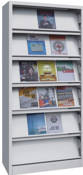
MY-SF-04 H1850*W900*D400mm
